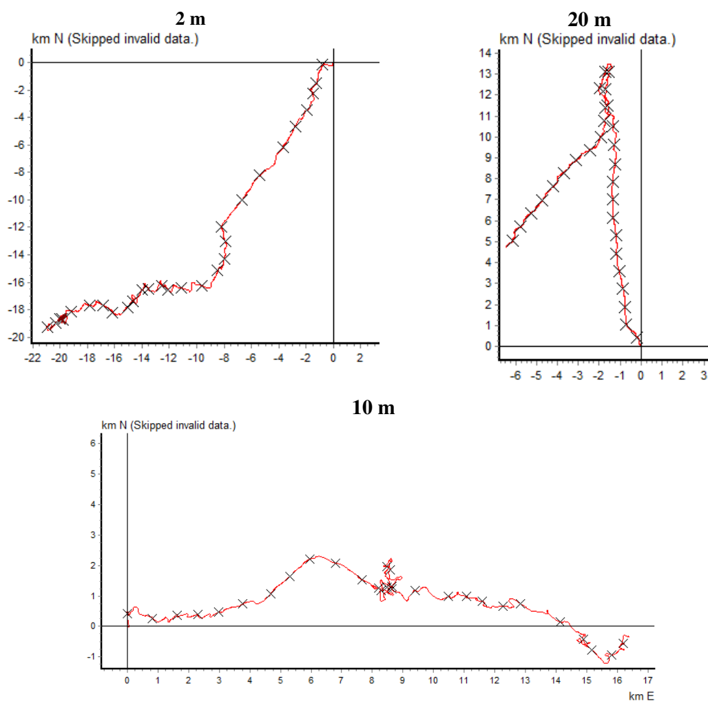
Figur 12. Progressivt vektorplott for målingene på 2 og 20 m dyp (oppe til venstre og høyre) og 10 m dyp (nede) i sjøområdet utenfor Nesfossen i perioden 12. mars – 10. april 2013.
