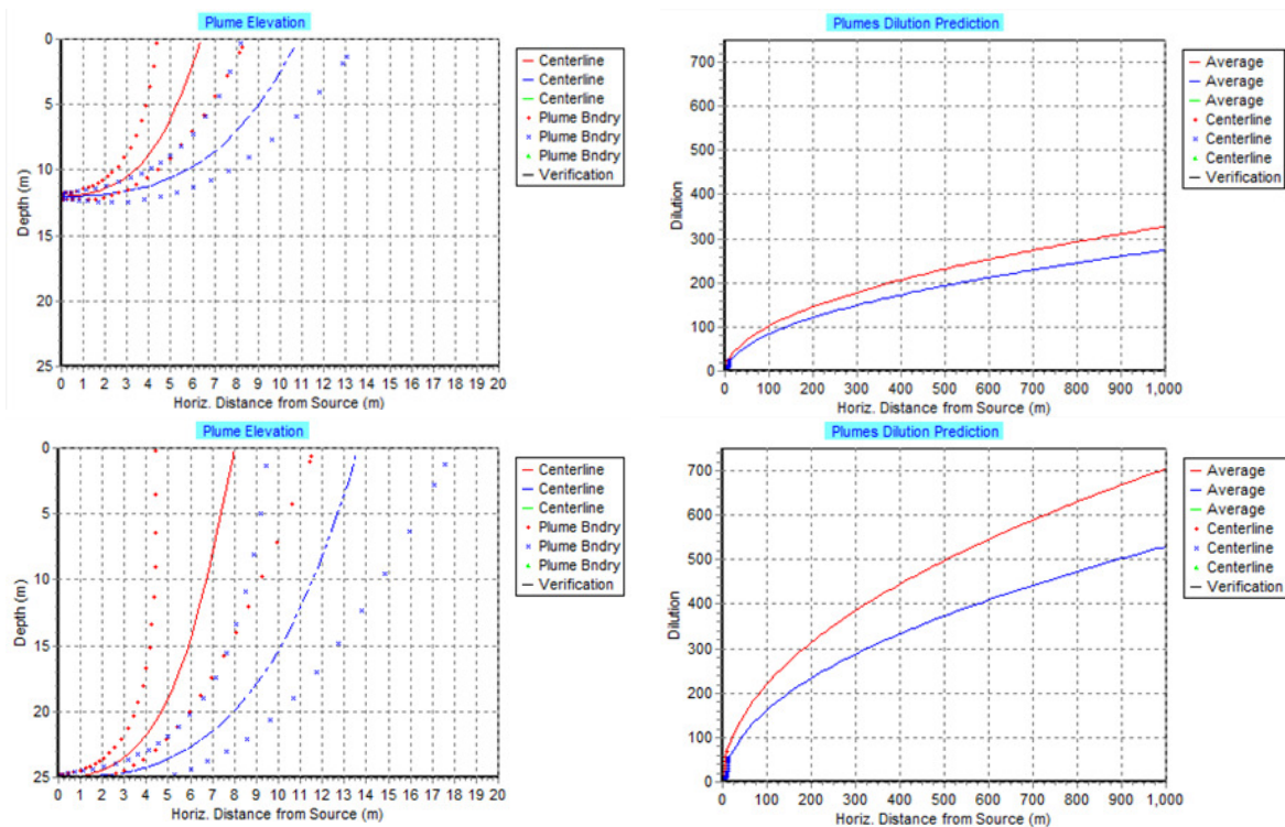
Figur 25. Nesfossen. Innlagringsdyp og fortykning ved et utslipp på 13 m dyp ved midlere (rød linje) og maksimal (blå linje) vannføring (øverst til venstre og høyre) samt ved et utslipp på 25 m dyp ved midlere (rød linje) og maksimal (blå linje) vannføring (nederst til venstre og høyre) for en typisk vintersituasjon. Figuren viser "strålebanene" for de to vannmengdene ved midlere strømhastighet. Utslippene som ligger på 12 m dyp har gjennomslag til overflaten (til høyre).
