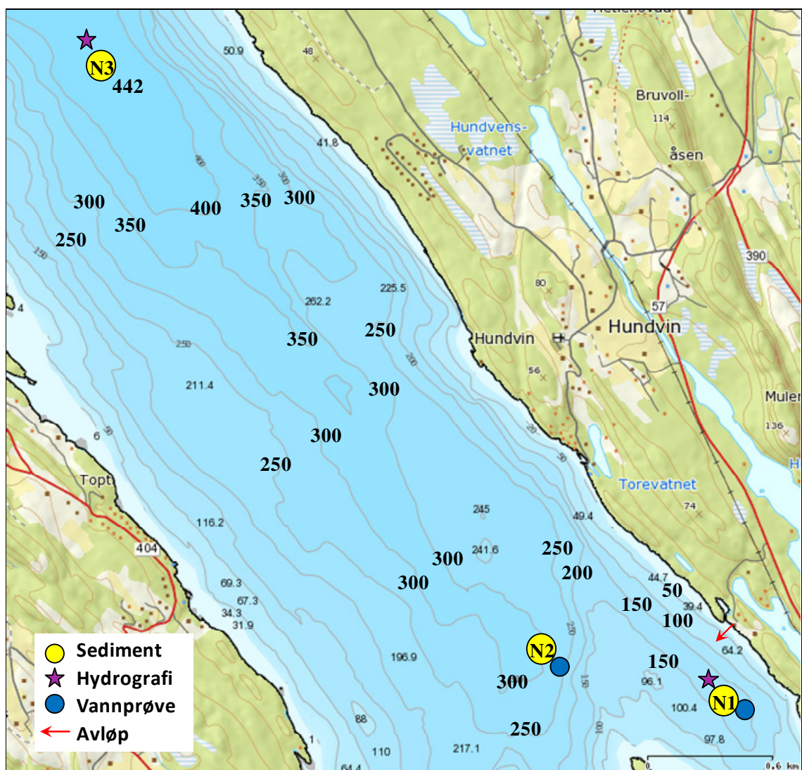
Figur 4. Stasjonene NES 1 – NES 3 i MOM C-resipientundersøkelsen av sjøområdene utenfor avløpene fra Nesfossen Smolt AS 12. mars 2013.
