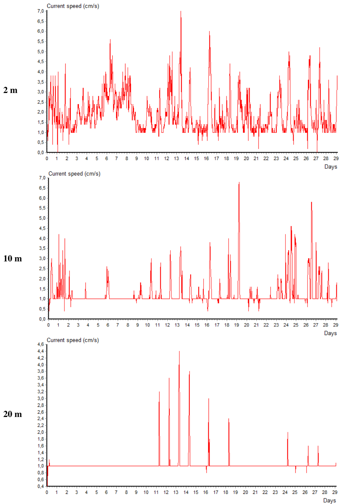
Figur 9. Strømhastighet i sjøområdet utenfor Nesfossen på 2, 10 og 20 m dyp i perioden 12. mars – 10. april 2013.
