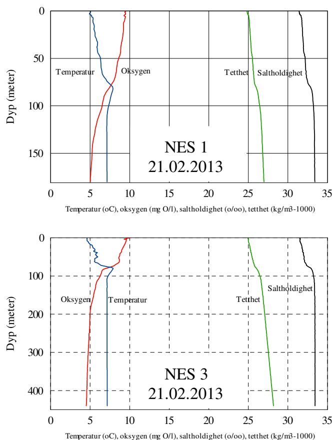
Figur 6. Temperatur-, saltinnhold- og oksygenprofiler på stasjonene NES 1 og NES 3 i Lurefjorden målt den 21. februar 2013.
