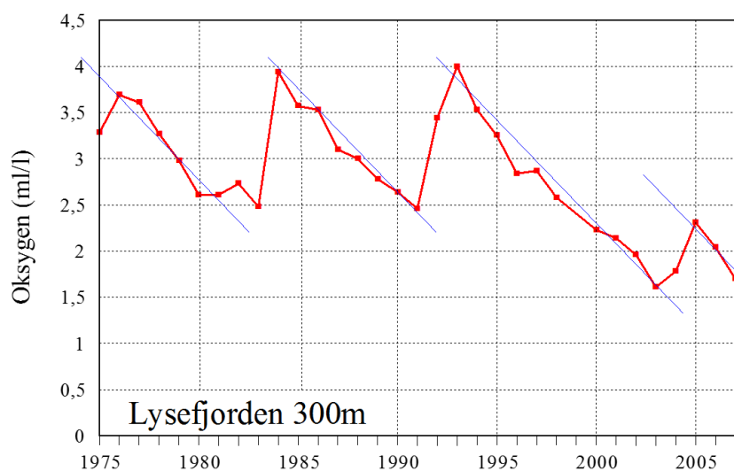
Figur 19. Årlige målinger av oksygeninnhold i bassengvannet på 300 m dyp i Lysefjorden i Rogaland mellom 1975 og 2007. Blå linjer viser konstant oksygenfor-bruksrate på 0,02 ml/l/mnd. Oksygendata fra Havforskningsinstituttets måleserie (stilt til rådighet av Jan Aure for Johnsen m.fl. 2008).
