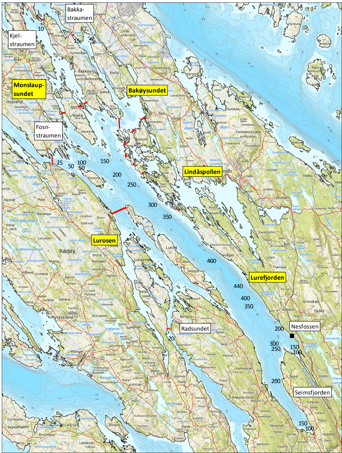
Figur 2. Enkelt dybdekart over Lurefjordenbassenget med inndeling av vannforekomster etter Fjordkatalogen, og plassering av terskler og terskeldyp samt anlegget og utslippet utenfor Nesfossen (fra http://kart.fiskeridir.no/adaptive/ ).
