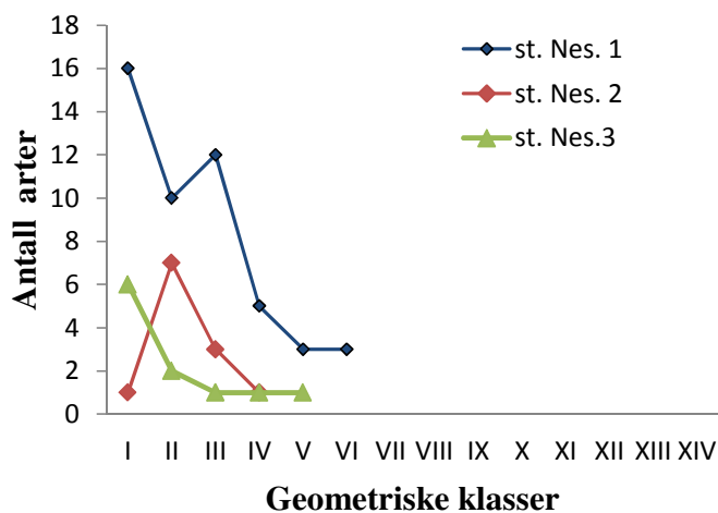
Figur 15. Faunastruktur uttrykt i geometriske klasser for stasjonene NES 1 – NES 3 i Kråkeosen og Lurefjorden 12. mars 2013. Antall arter langs y-aksen og geometriske klasser langs x-aksen
