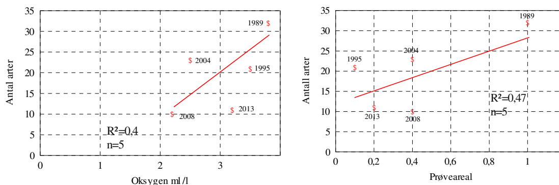
Figur 22. Sammenheng mellom variasjon i antall arter og oksygenforhold (til venstre) og prøvearealets størrelse (til høyre) ved det dypeste i Lurefjorden i perioden 1989 – 2013.
