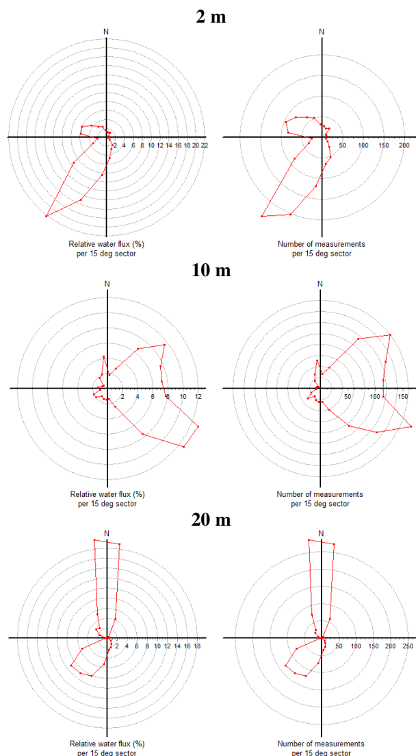
Figur 11. Strømroser som viser fordelingen av henholdsvis vanntransport og antall målinger (strømretning) for hver 15. grad for måleresultatene i sjøområdet utenfor Nesfossen på 2, 10 og 20 m dyp i perioden 12. mars – 10. april 2013.
