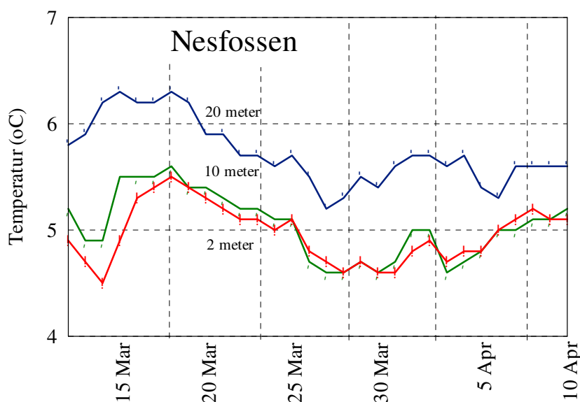
Figur 5. Døgnmidler for temperatur målt på 2 m dyp (rød strek), 10 m dyp (grønn strek) og 20 m dyp (blå strek) utenfor Nesfossen i perioden 12. mars – 10. april 2013.
