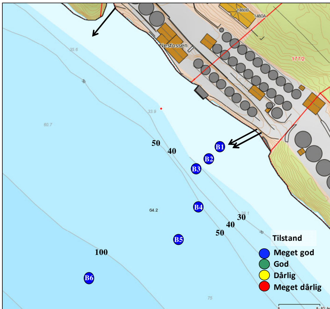
Figur 17. Oversikt over MOM B-tilstand (middelverdien av gruppe II og III parametre) for de seks grabbhoggene som ble tatt utenfor avløpene på Nesfossen 21. februar 2013 (jf. tabell 19 ).
