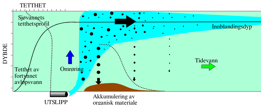
Figur 24. Prinsippskisse for primærfortynningsfasen av innblanding av et ferskvannsutslipp i en sjøresipient, med gjennomslag til overflaten og kun lokal sedimentering av organiske tilførsler i resipientens umiddelbare nærhet til utslippspunktet. Utslippet får økt sin tetthet ettersom det lettere ferskvannet stiger opp og blandes med sjøvannet (heltrukken linje og lyseblått).
