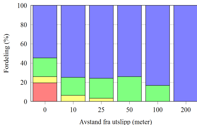
Figur 26. Sammenstilling av resultater fra Rådgivende Biologer AS 31 undersøkelser av utslipp til sjø fra settefiskanlegg, der det er benyttet MOM-B / NS 9410:2007-metodikk med grabbhogg i økende avstand fra selve utslippspunktet. Fargene er i henhold til NS 9410:2007: Blå = "meget god", grønn = "god", gul = "dårlig" og rød = "meget dårlig" miljøtilstand
