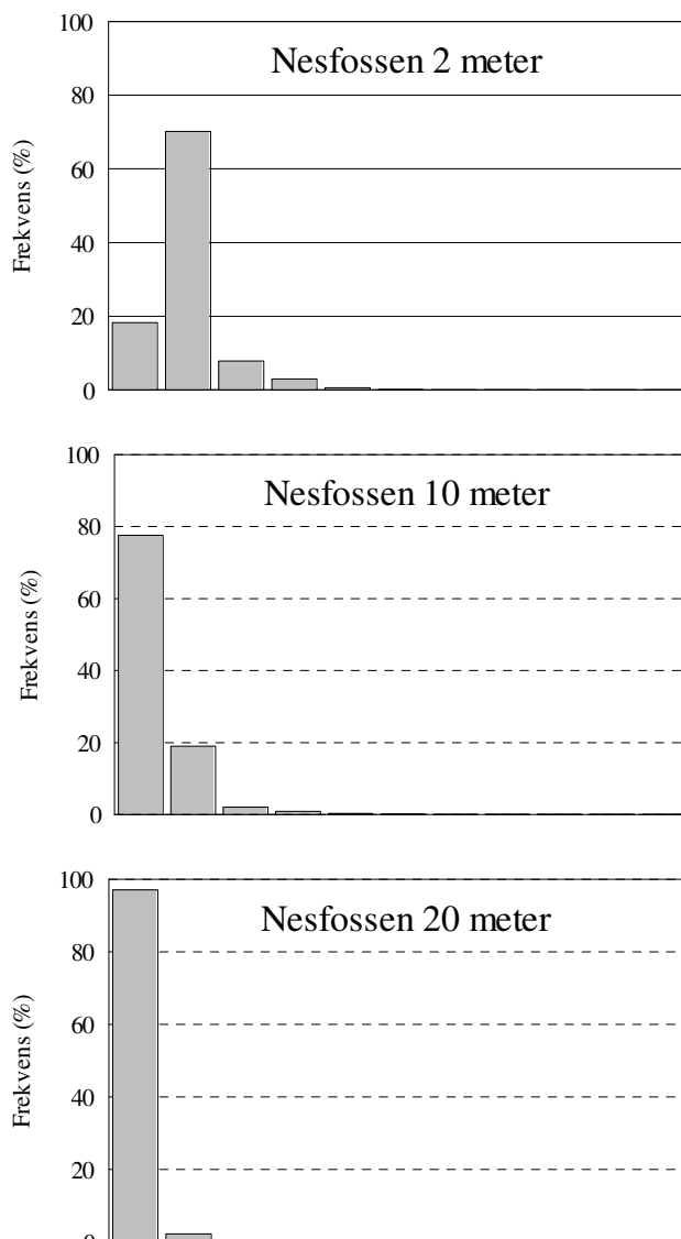
Figur 8. Fordeling av strømhastighet i sjøområdet utenfor Nesfossen på 2, 10 og 20 m dyp i perioden 12. mars – 10. april 2013.
