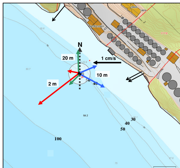
Figur 7. Målt hovedstrømretning og strømfart på de ulike måledypene i sjøområdet utenfor Nesfossen like utenfor avløpene til settefiskanlegget.
