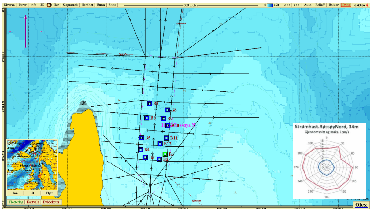
Figur 2 Dybdekart ved Røssøya N. Prøvetakingsstasjonene er tegnet inn med fargekode som beskriver tilstand iht NS 9410:2016 (1 = blå, 2 = grønn, 3 = gul, 4 = rød). Strømrøse i høyre hjørne viser retning av vanntransport ved spredningsmåling (34 m) på lokaliteten (Argus Miljø v/Morten Krogstad).
