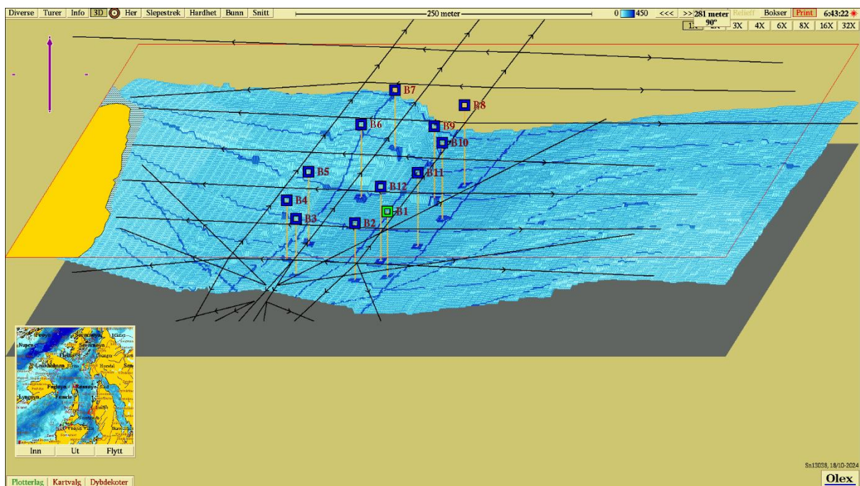
Figur 3. 3D visning av bunntopografi ved Røssøya N med nummererte stasjoner gjengitt i Figur 2
